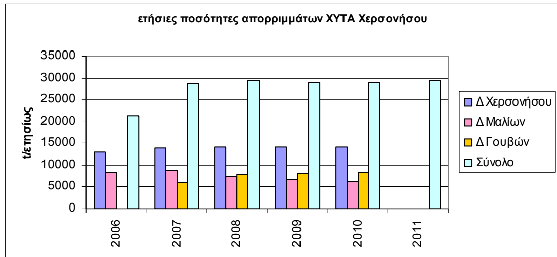
Διάγραμμα 18: Ποσότητες απορριμμάτων που δέχεται ο ΧΥΤΑ ΦΟΔΣΑ Β. Πεδιάδος ετησίως.
