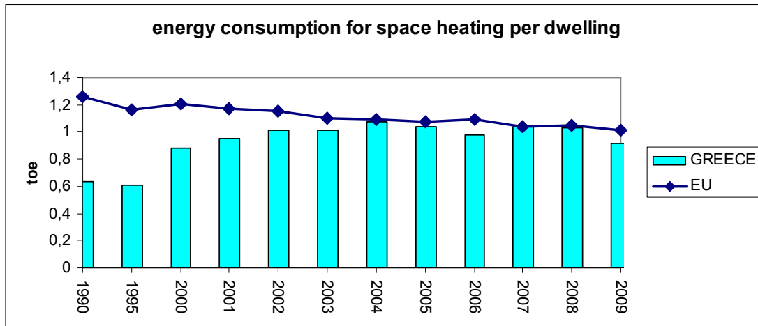
Διάγραμμα 22: Ενεργειακή Κατανάλωση για θέρμανση ανά κατοικία στην Ελλάδα & Ε.Ε. 1990-2009.
