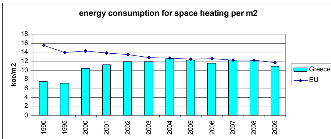
Διάγραμμα 23: Ενεργειακή Κατανάλωση για θέρμανση ανά τετραγωνικό μέτρο, Ελλάδα & Ε.Ε. 1990-2009.
