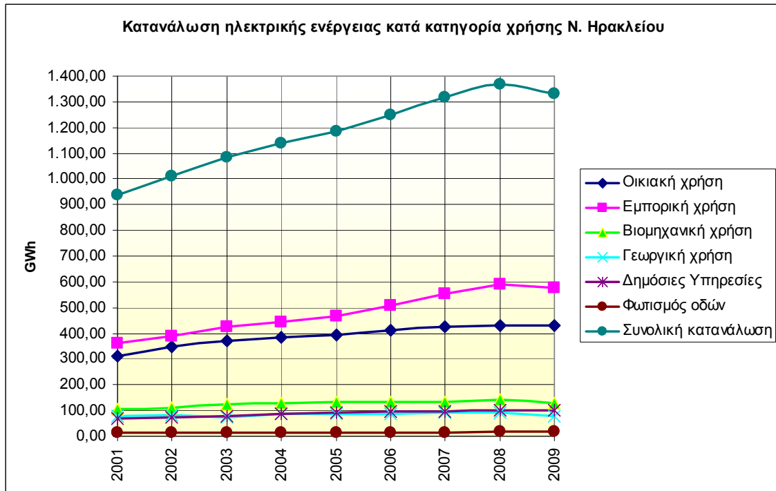
Διάγραμμα 29 : Ηλεκτρική κατανάλωση ανά τελική χρήση στο Ν. Ηρακλείου (2001-2009).
