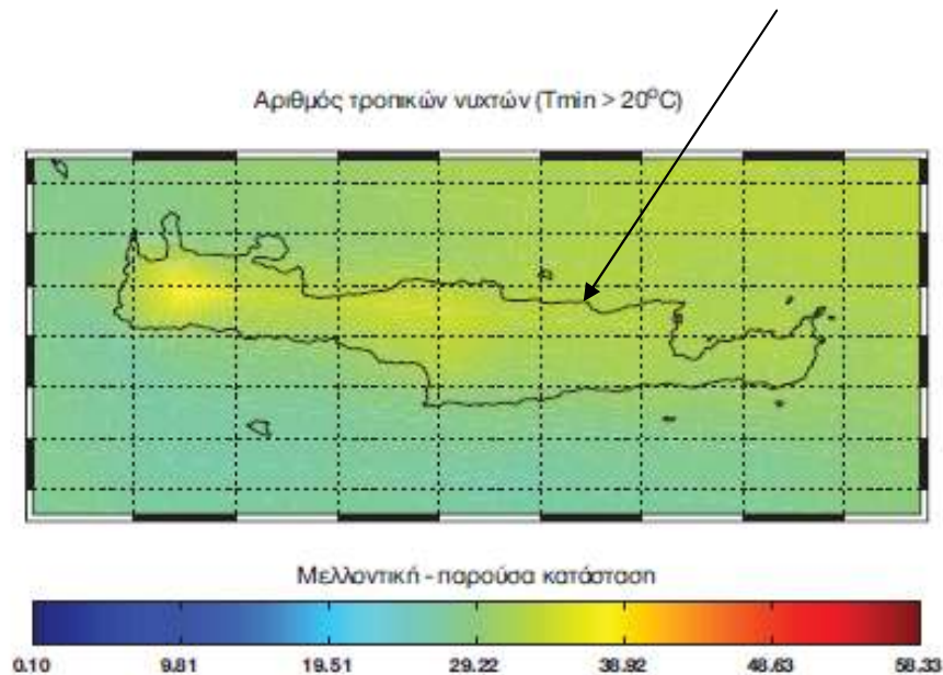
Εικόνα 5: Αριθμός τροπικών νυχτών ( T_{min} > 20^{\circ}\text{C} )
