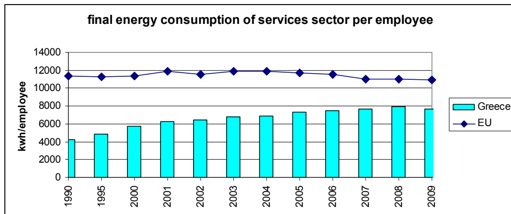
Διάγραμμα 16: Τελική Ενεργειακή κατανάλωση τομέα υπηρεσιών, ανά υπάλληλο στην Ελλάδα και Ε.Ε (1990-2009).
