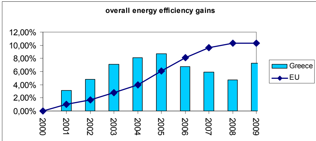
Διάγραμμα 8. Συνολική Ενεργειακή Αποδοτικότητα Ελλάδας – Ε.Ε. 2000-2009. Πηγή: http://www.odyssee-indicators.org/
