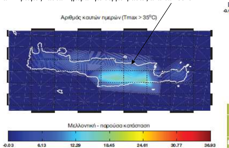
Εικόνα 4: Αριθμός καυτών ημερών με θερμοκρασίες άνω των 35°C
