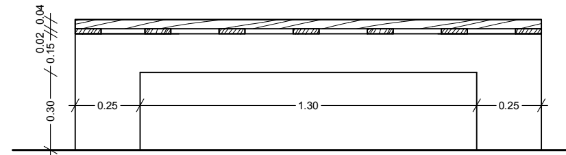
όψη
